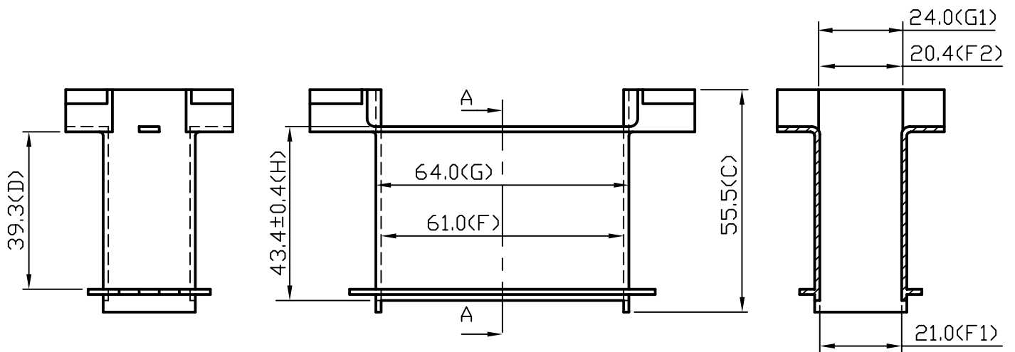
SECTION A-A
