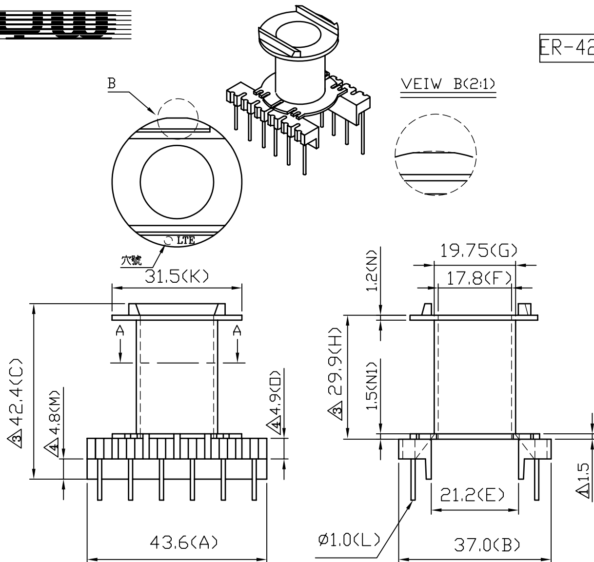
SECTION A-A
