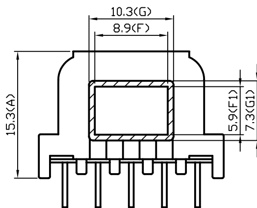
SEC A-A'
