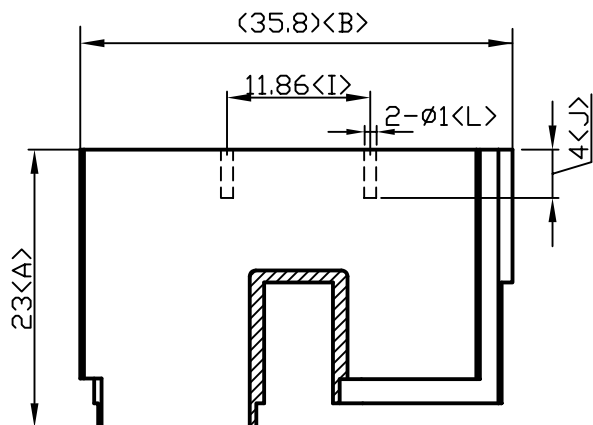
A-A VIEW
