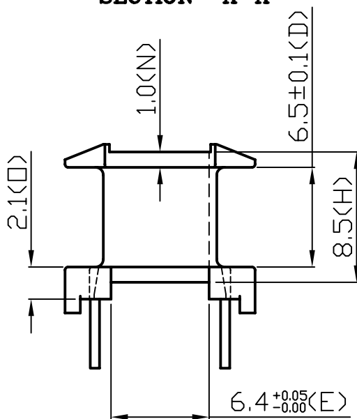
SECTION A-A
