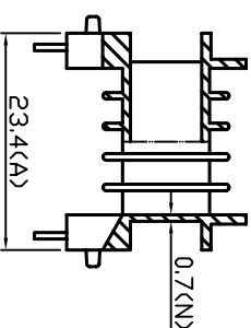
SECTION D-D
